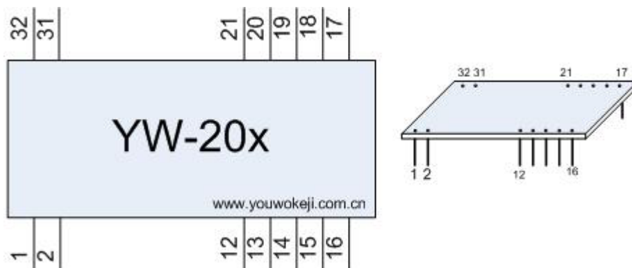
图 1 YW-204 引脚图
