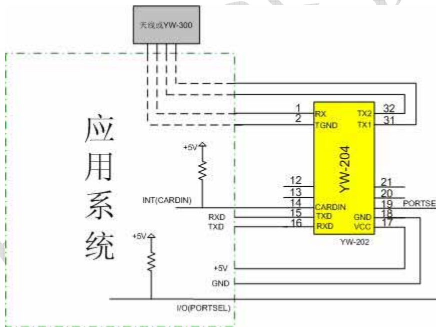
图 3 YW204 应用电路
