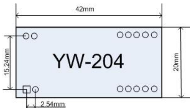
图 2 YW-204 封装图
